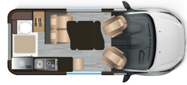
CAP LAND2 63 100 CHF Länge: 5,34 m Höhe: 2,00 m Breite: 1,99 m 4 Sitzplätze* / 2 + 2 Schlafplätze
